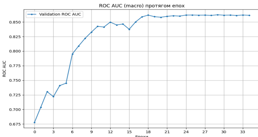
Рис. 2. Динаміка метрики ROC AUC (macro) протягом епох навчання
