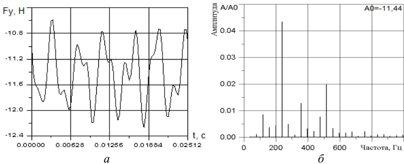
Рис. 4. Изменение аэродинамической силы, действующей на рабочую лопатку венца турбины (МЛФУ=+90 град): a – окружная сила; б – амплитудно-частотная характеристика
