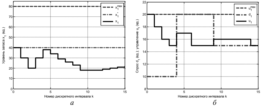
Рис. 2. Графики переходных процессов для узла 1 сети поставок
